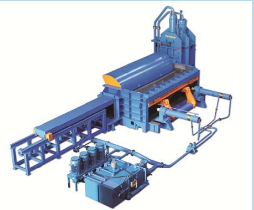
1250TON スクラップ プレス シャー(切断機)
